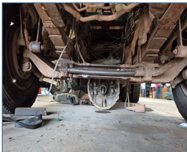
IMAGEM DO CAMINHÃO JÁ COM SEU MOTOR DESMONTADO NO DIA DA INSPEÇÃO
