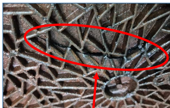
IMAGENS DO CÁRTER DANIFICADO QUE, AO TRINCAR, CAUSOU A PERDA DE ÓLEO, RESULTANDO EM FALTA DE LUBRIFICAÇÃO E DANOS DIRETOS AO MOTOR
